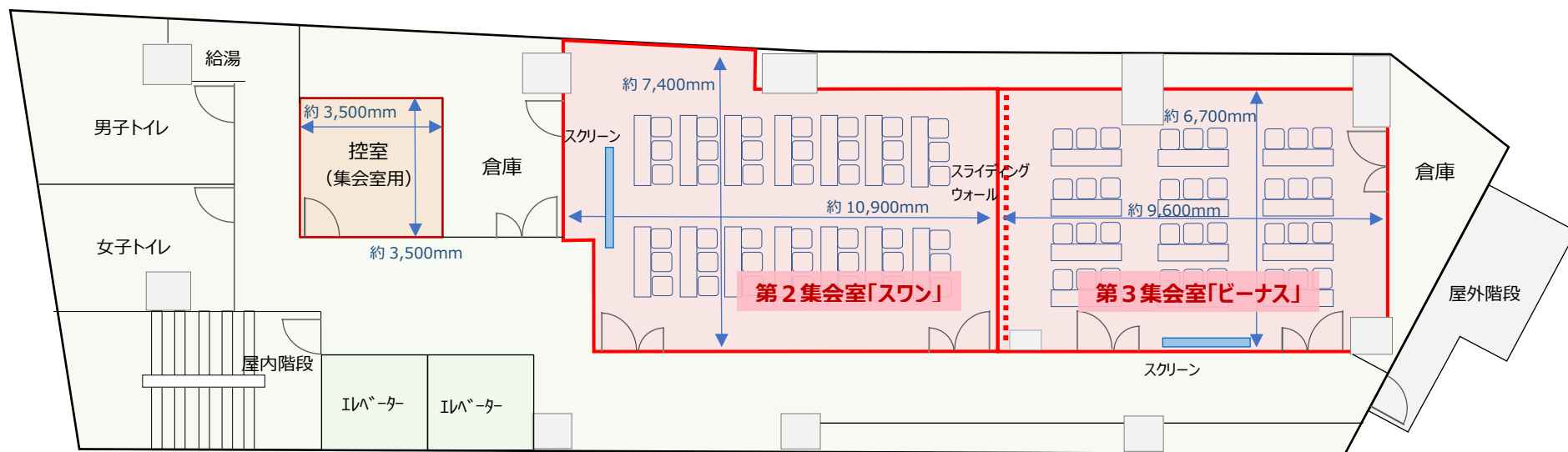
【6階平面図】
